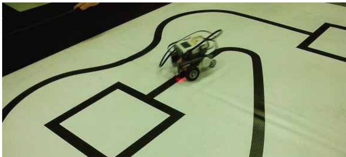
1、單光循跡:循跡沿著黑線邊緣前進到達終點。
