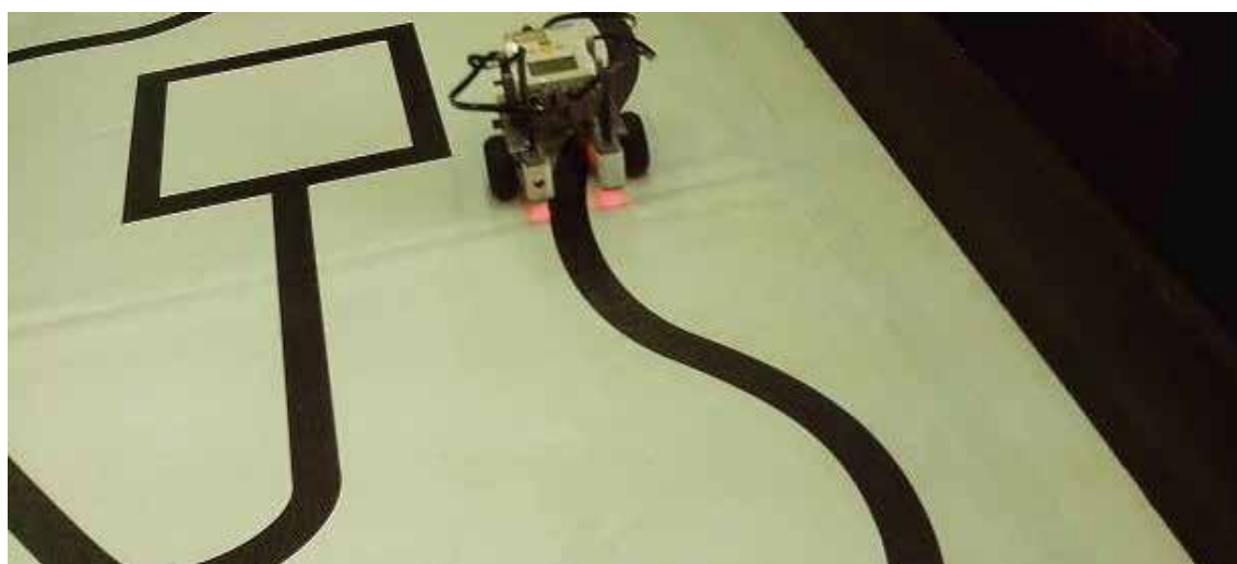
2、雙光循跡:雙光機器人從黑色起跑線出發沿著黑線到達黑色終點線。
