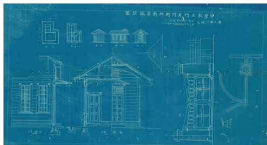
校門建設
