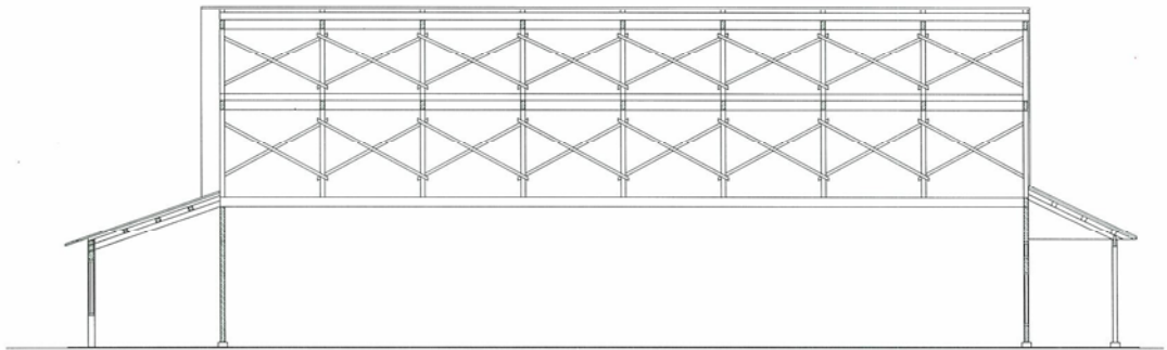
北向剖立面圖
