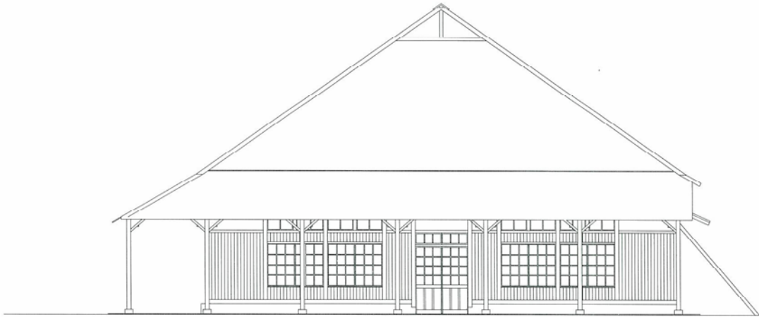
西向立面圖
