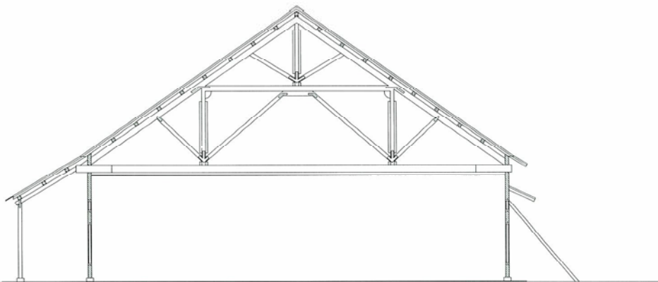
101 西向剖立面圖（禮堂部份）
