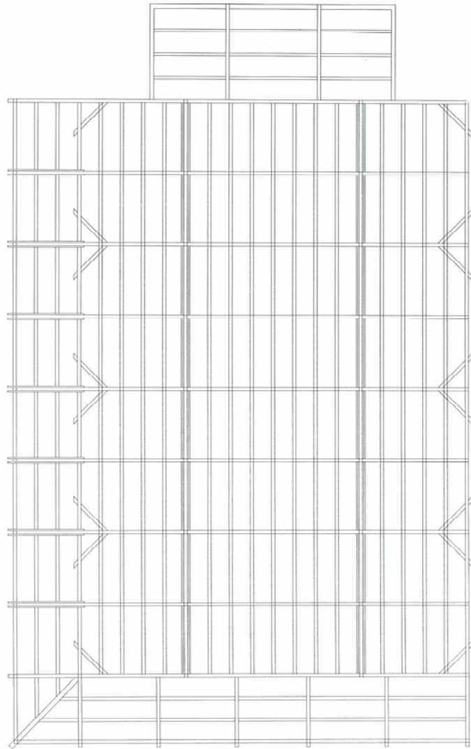
屋頂架平面圖
