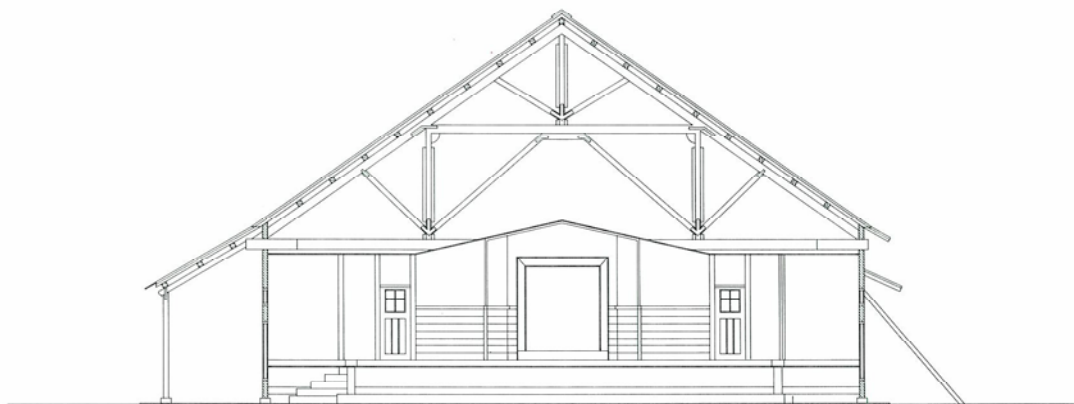
西向剖立面圖（講台部份）
