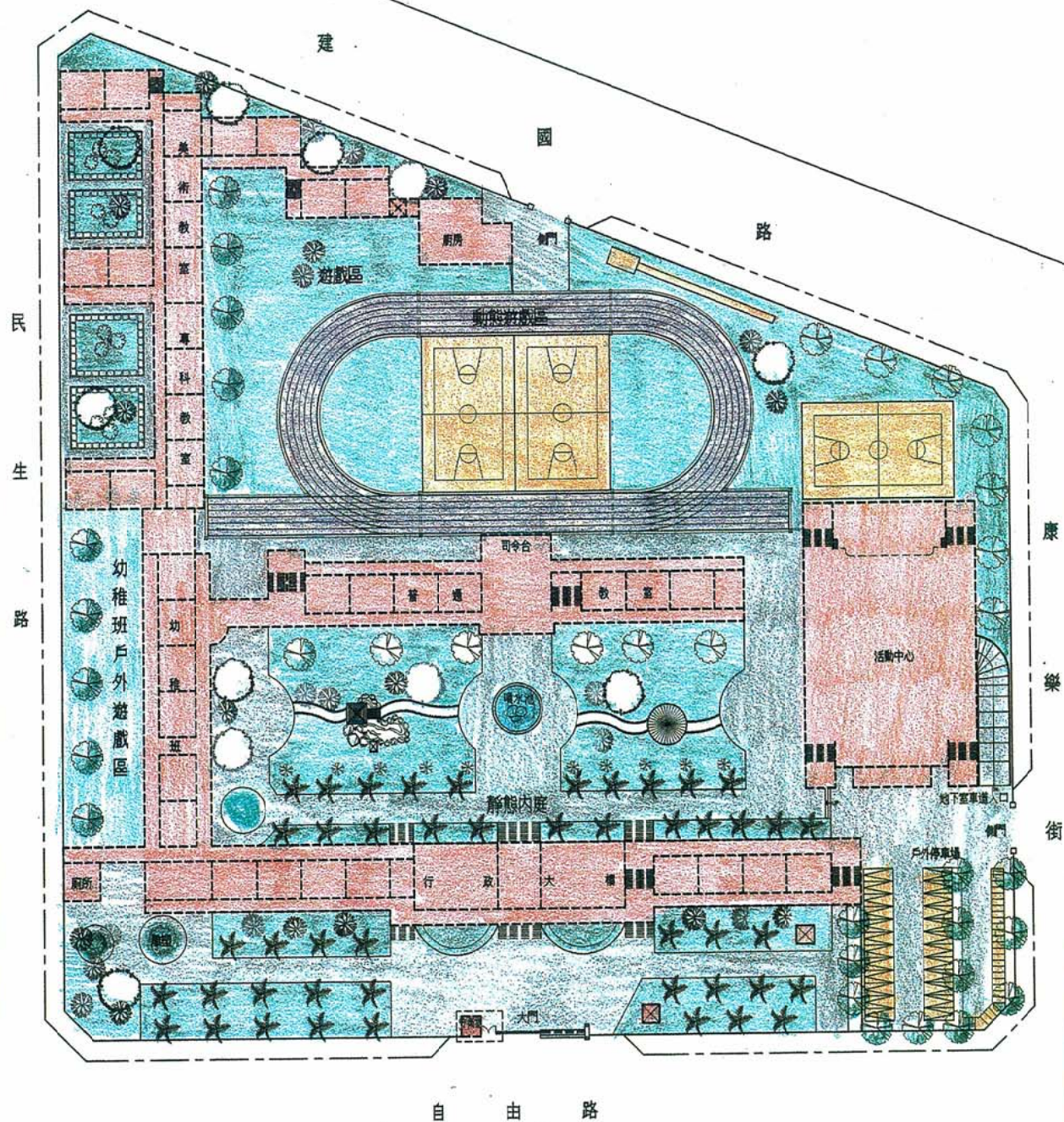
台中市大同國小校園規劃配置圖 S=1/600 (A案)
