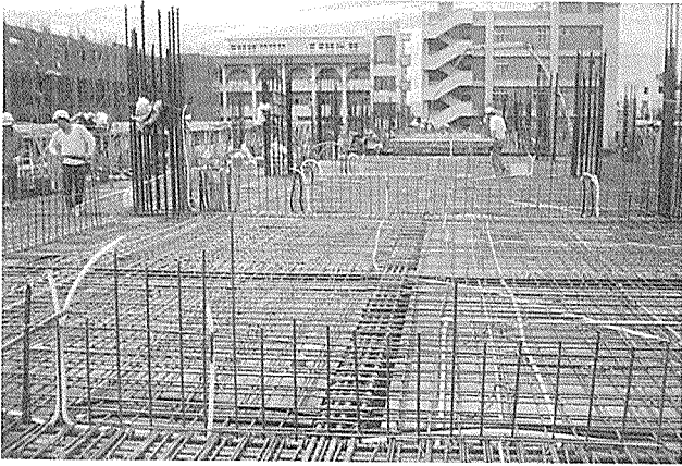
〈樓板鋼筋組立完成〉
