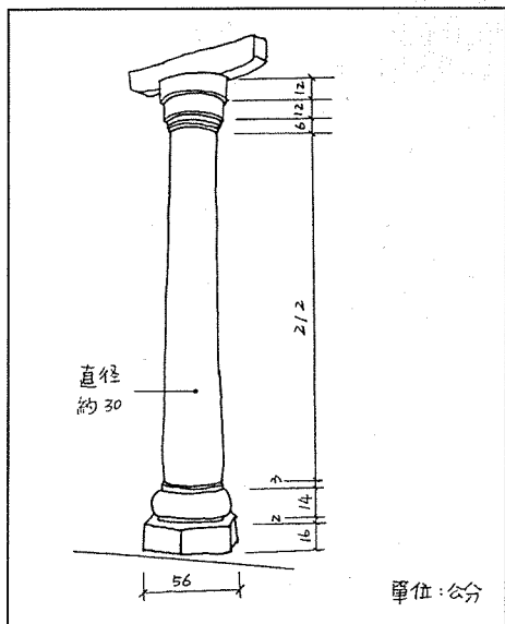
圖二 冂字形北側教室立面示意圖 蔡紹斌 / 繪
